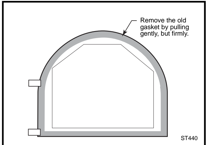
Fig. 27 Door gasket.
